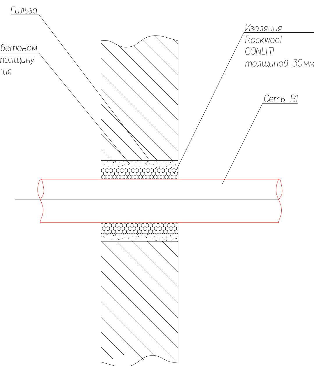
Узел прохода сетей через перегородку
